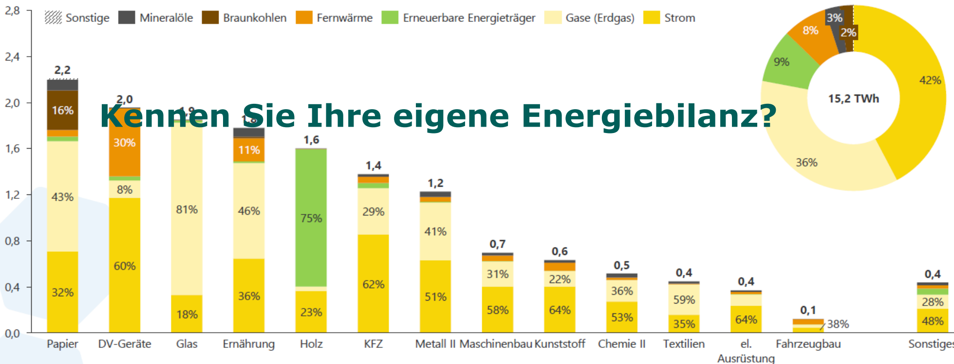
Endenergieverbrauch ausgewählter Branchen in TWh | Sachsen | 2022
